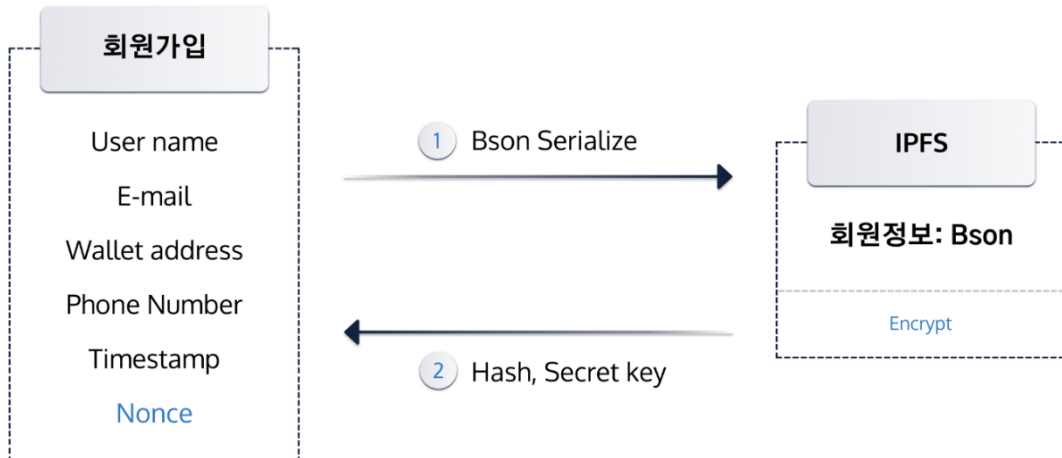
[ 그림 38 ] 공동인증시스템 구조도
