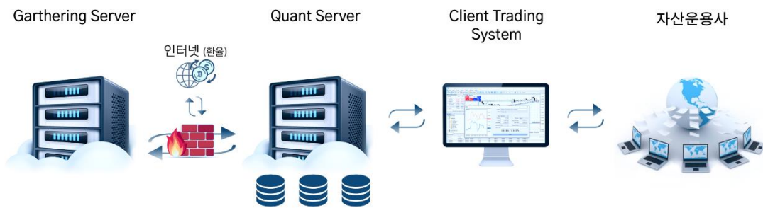
[그림 15] Quant Trading System 구조
