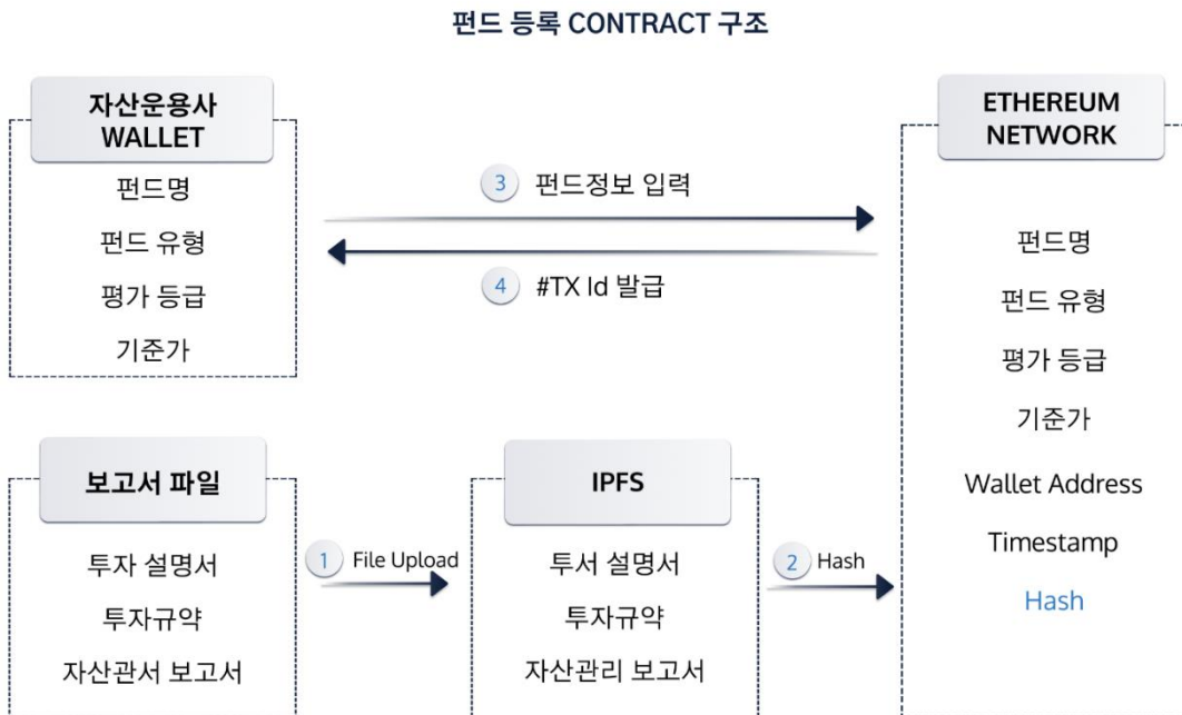
[ 그림 35 ] 펀드 등록 CONTRACT 구조도
