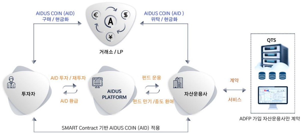
[ 그림 27 ] ADFP 기반 탈중앙화 펀드마켓 운영 구조
